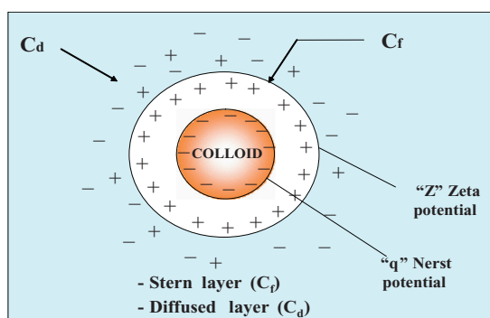
Fig. 1. Flocculant destabilisation.
